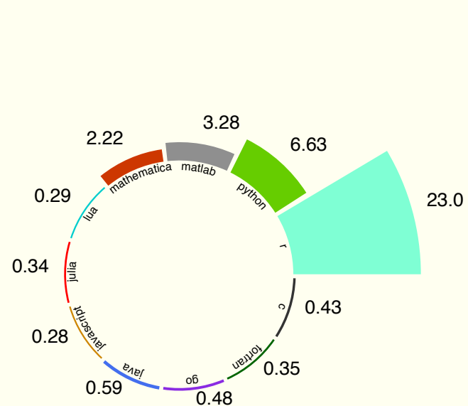
mandel
