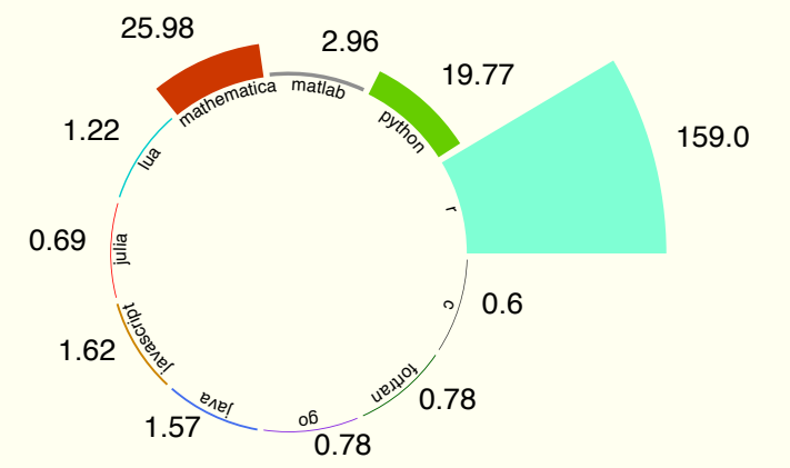
quicksort
