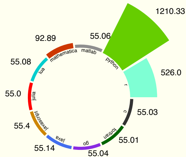
pi_sum
