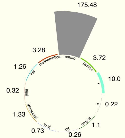
parse_int
