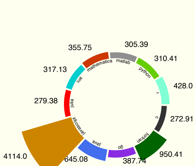
rand_mat_mul
