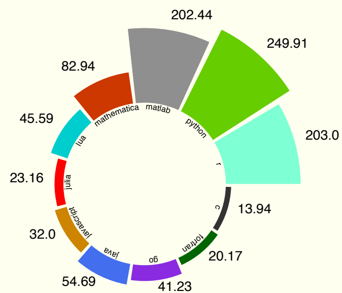
rand_mat_stat
