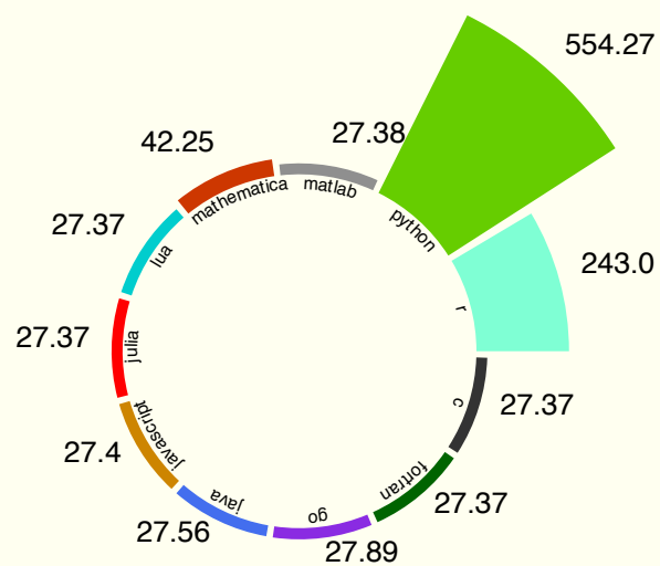
iteration_pi_sum
