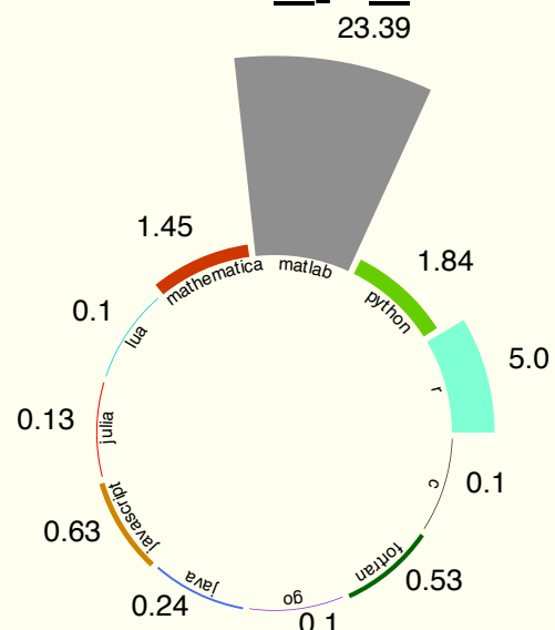
iteration_pi_sum
