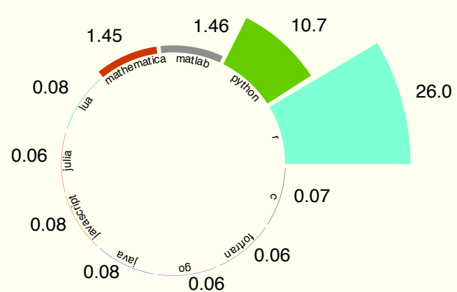
userfunc_mandelbrot
